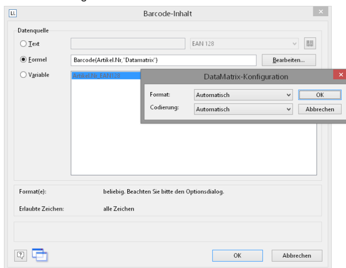
Abbildung 13.10: Barcodeoptionen
