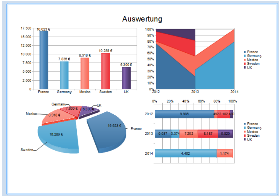
Abbildung 6.71: Mehrspätiger Berichtscontainer
