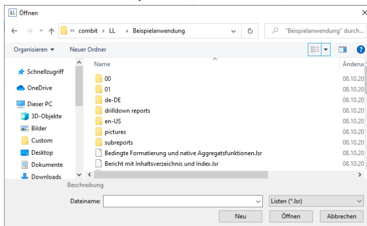
Abbildung 2.2: Öffnen-Dialog
