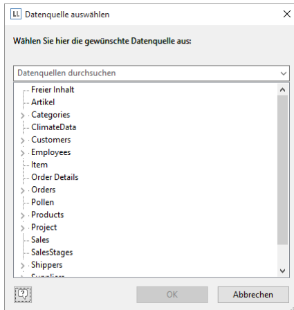
Abbildung 5.11: Datenquelle auswählen
