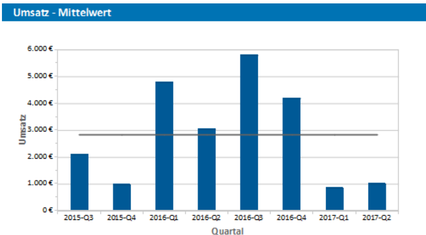
Abbildung 6.28: Mittelwertgerade
