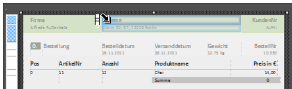
Abbildung 3.12: Spalte selektieren
