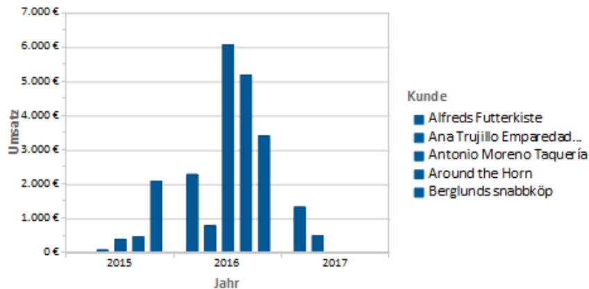
Abbildung 6.8: Gruppierendes Balkendiagramm
