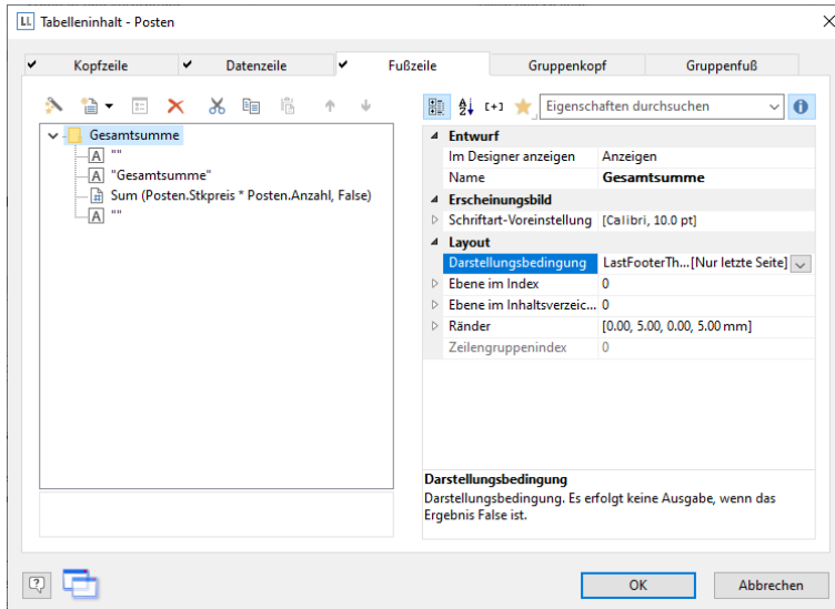
Abbildung 2.56: Darstellungsbedingung
