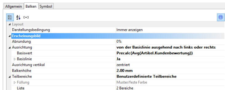
Abbildung 6.39: Balken-Eigenschaften
